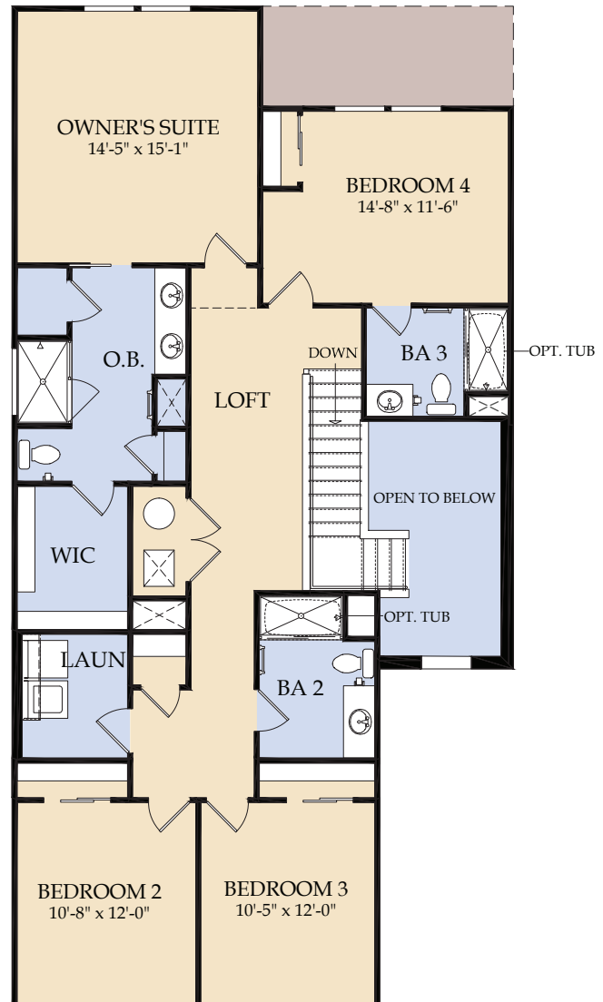
Segundo piso
