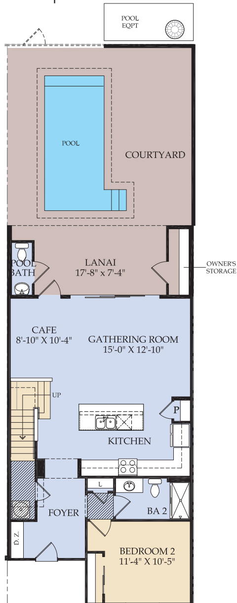
Primer piso
