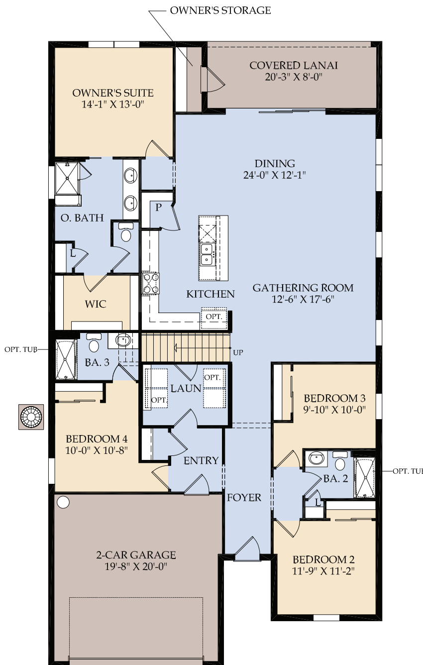
Primer piso
